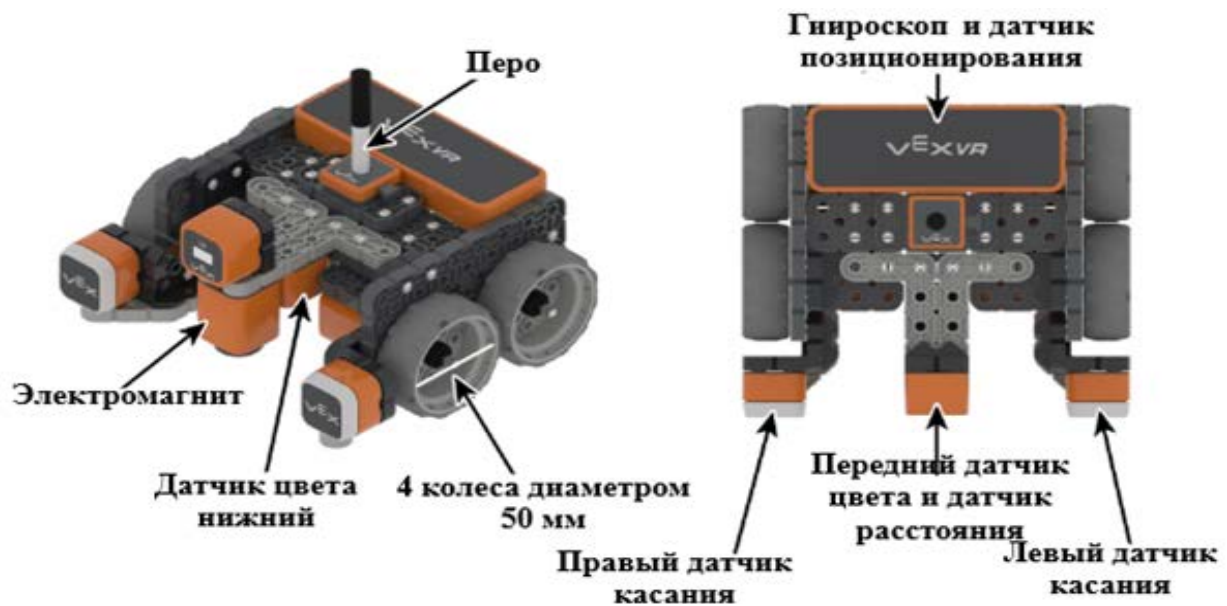
Рис. 7. Конфигурация датчиков робота
