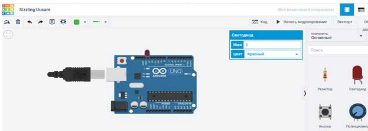
Рис. 163. Вид программы
