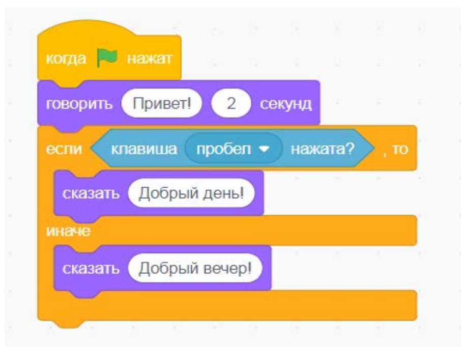
Рис. 122. Вид программы
