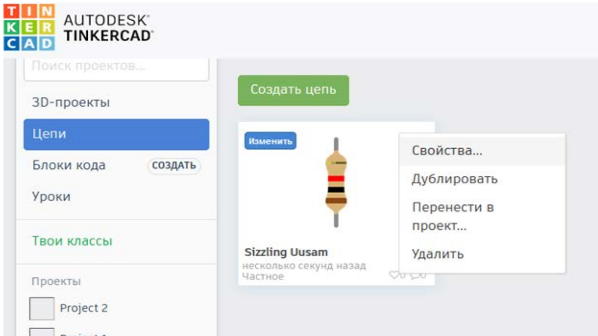
Рис. 162. Вид программы
